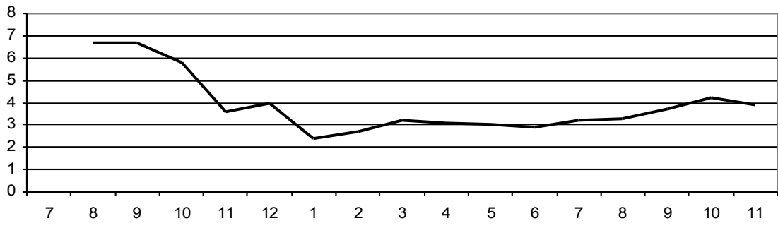
Рис. 2. Щомісячні обсяги експорту у 2008-2009 рр., млрд дол.
